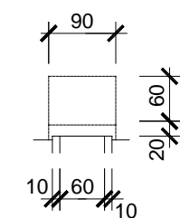
keresztmetszet
