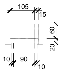
hosszmetszet
